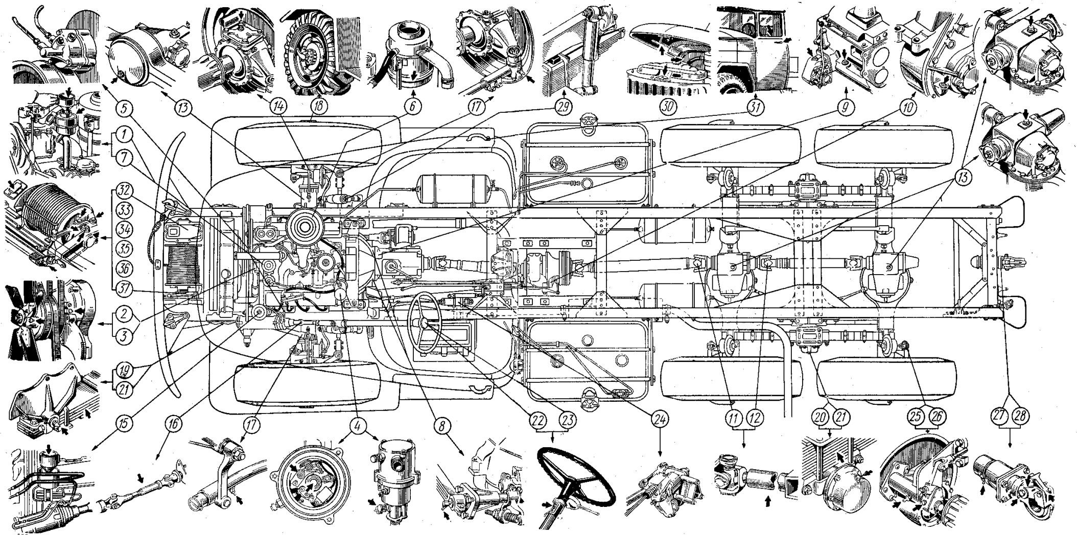
Рис. 122. Карта смазки автомобиля ЗИЛ-131
